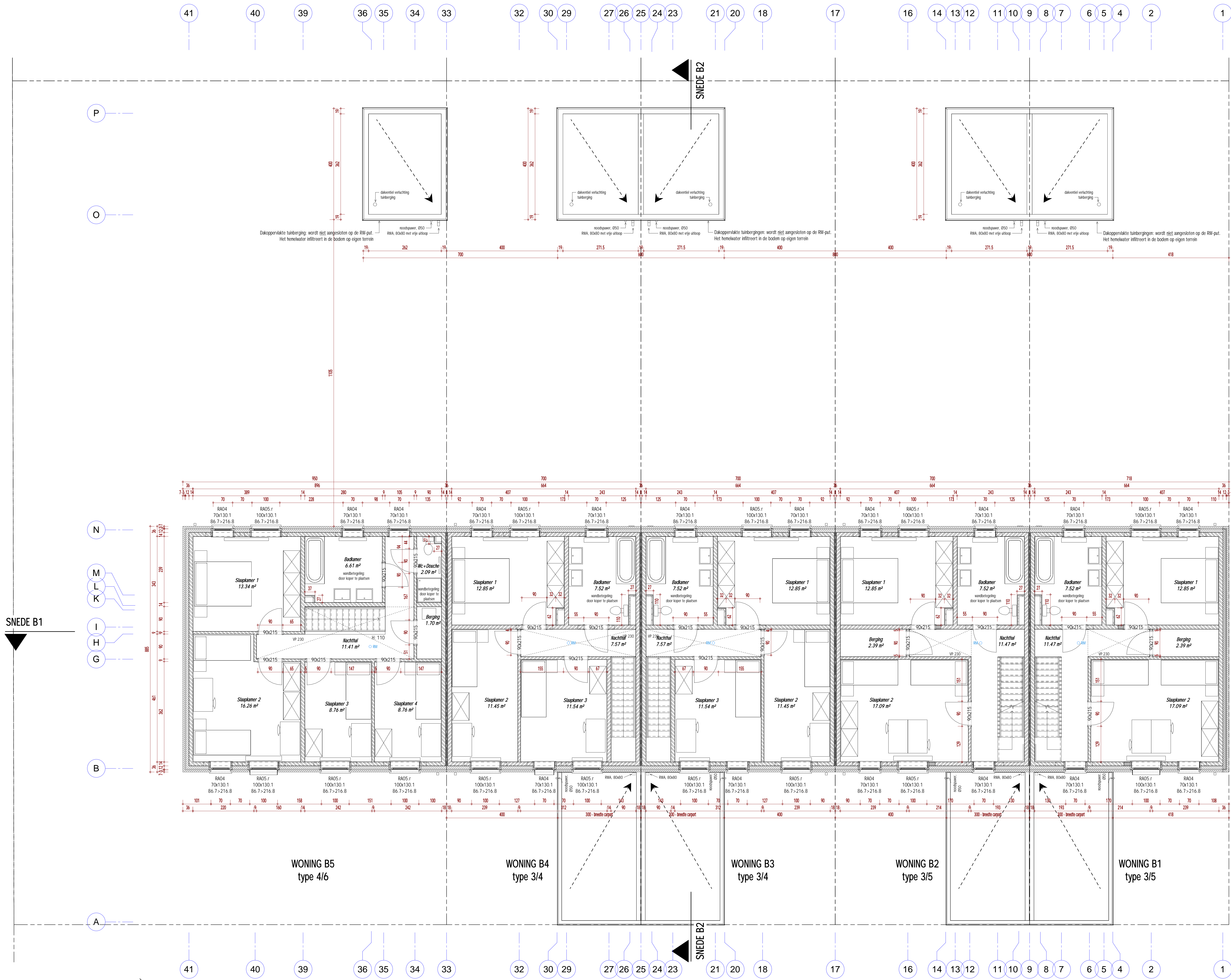
Schaal 1 : 50 1 Blok B - Verdieping 1
