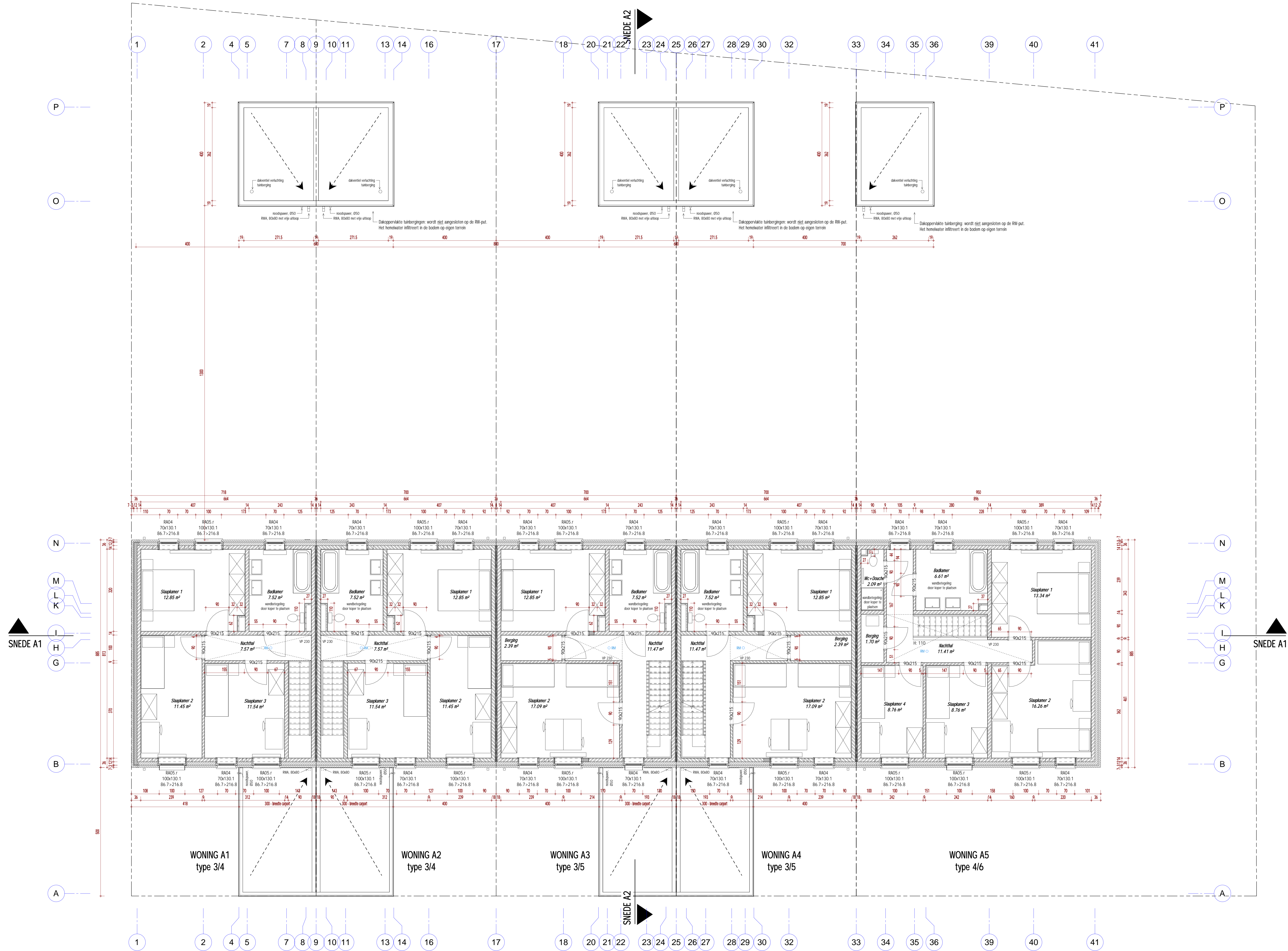
Schaal 1 - 50 1 Blok A - Verdieping 1
